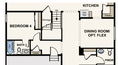
OPT. BEDROOM 4/BATH 3 SUITE
