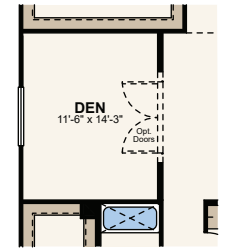
OPT. DEN ILO SUPER LOFT
