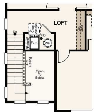
OPT. LOFT
